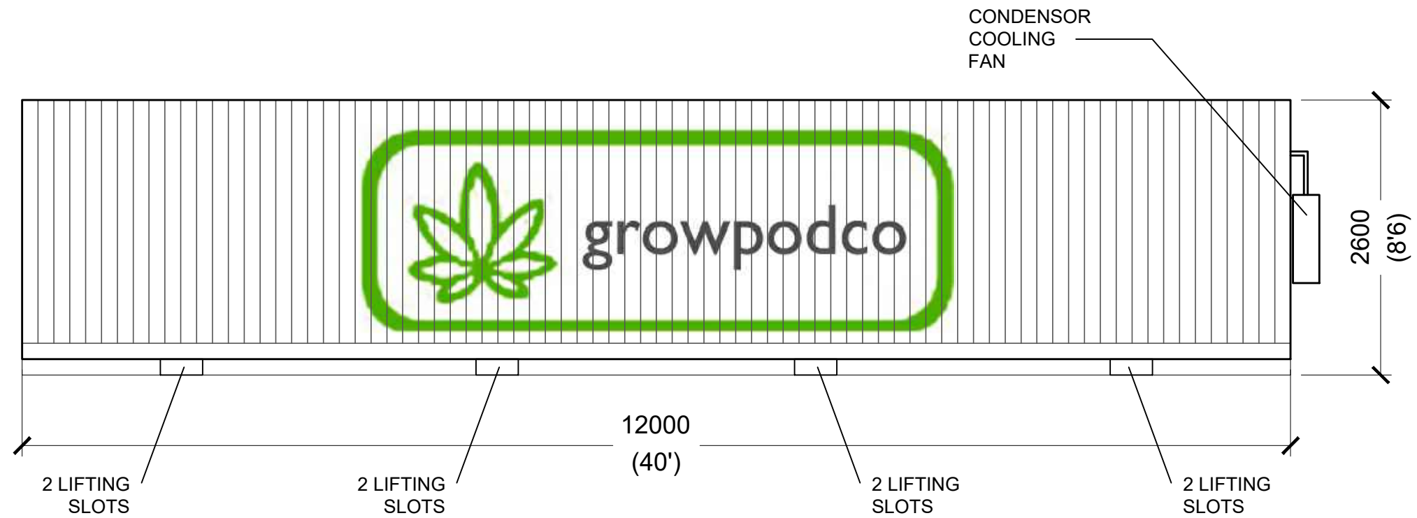
RIGHT ELEVATION
